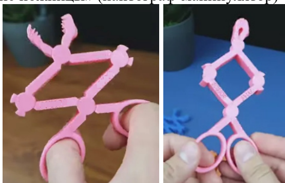
Рис.1.Образец и модель изделия «Телескопические ножницы» (пантограф-манипулятор)
